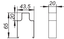
clé de maintenance pour caniveau de douche
